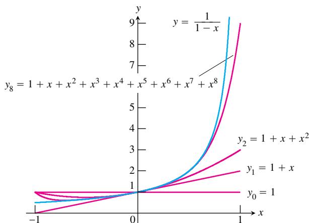
ΣΧΗΜΑ 8.16 Γραφικές παραστάσεις της f(x) = 1/(1 - x) και τεσσάρων πολυωνυμικών της προσεγγίσεων. (Παράδειγμα 1)
